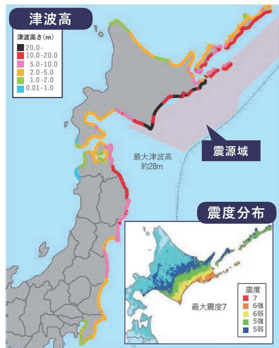
千島海溝沿いの地震
